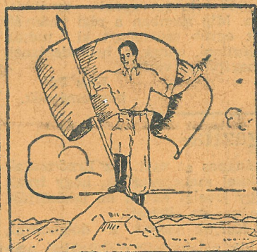
1. Ernő-mező
